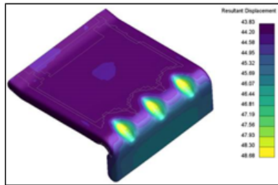
Viridis
